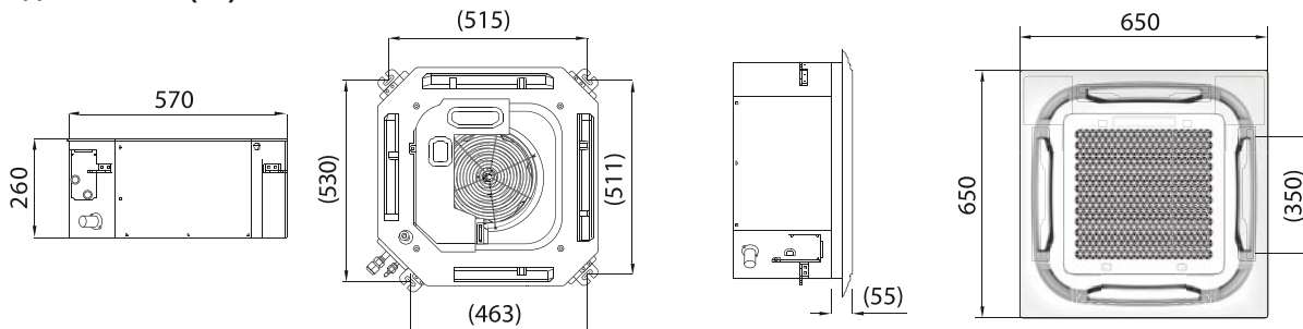
Модели QV-I24(36, 48, 60)CG
