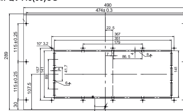
Модели QV-I48(60)CG
