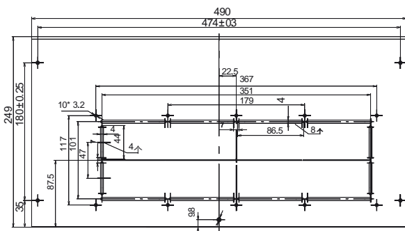
Модели QV-I24(36)CG
